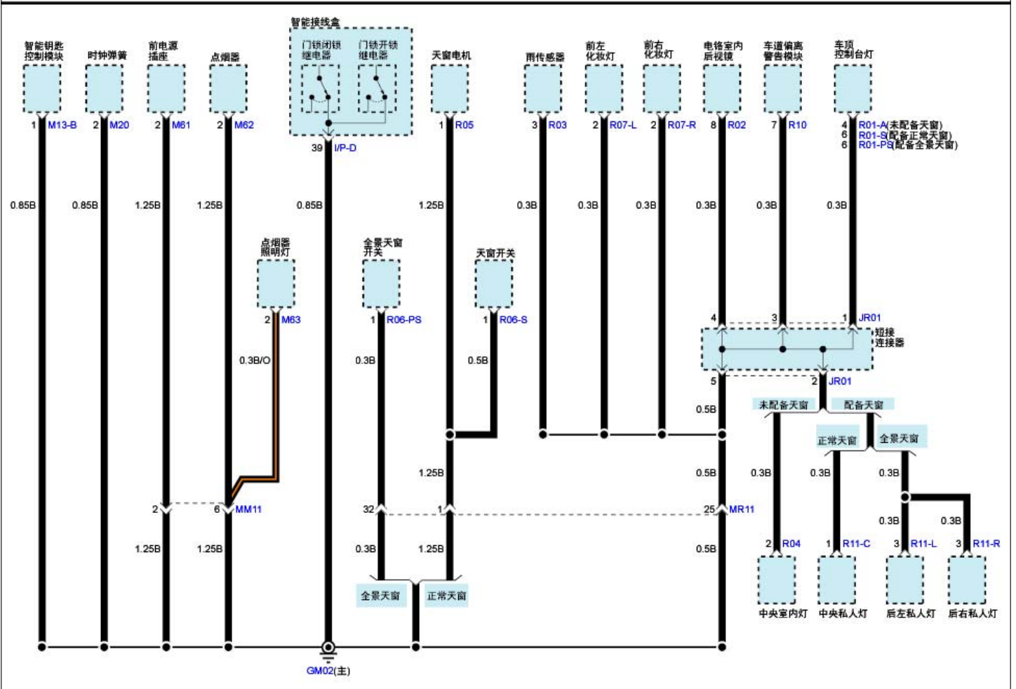
搭铁分布(3)
